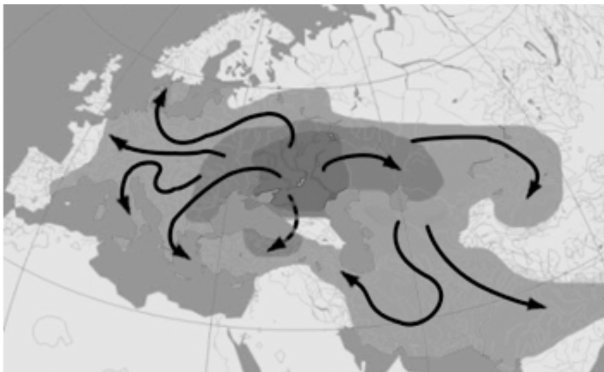
Рисунок 2. Индоевропейское расселение.
