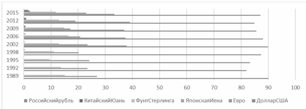
Рис. 4. Валютная структура оборота на рынке FOREX 1 [Сайт рынка Форекс, www]
