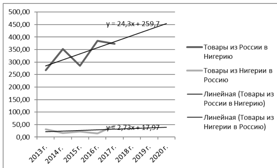
Рисунок 5 – Прогнозирование товарооборота России и Нигерии на основании линейного тренда
